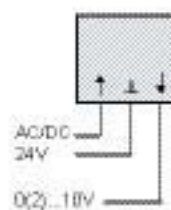
Posicionador PM/PT
