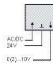
Posicionador PM/PT
